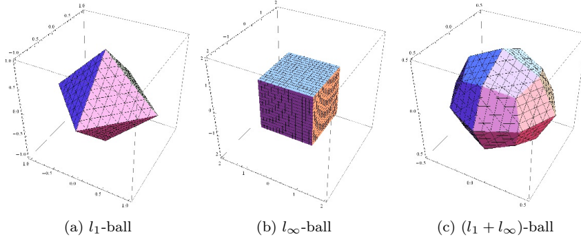
Fig. 2.1: l_1 + l_\infty norm
